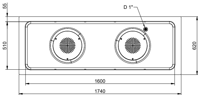
Boven aanzicht
